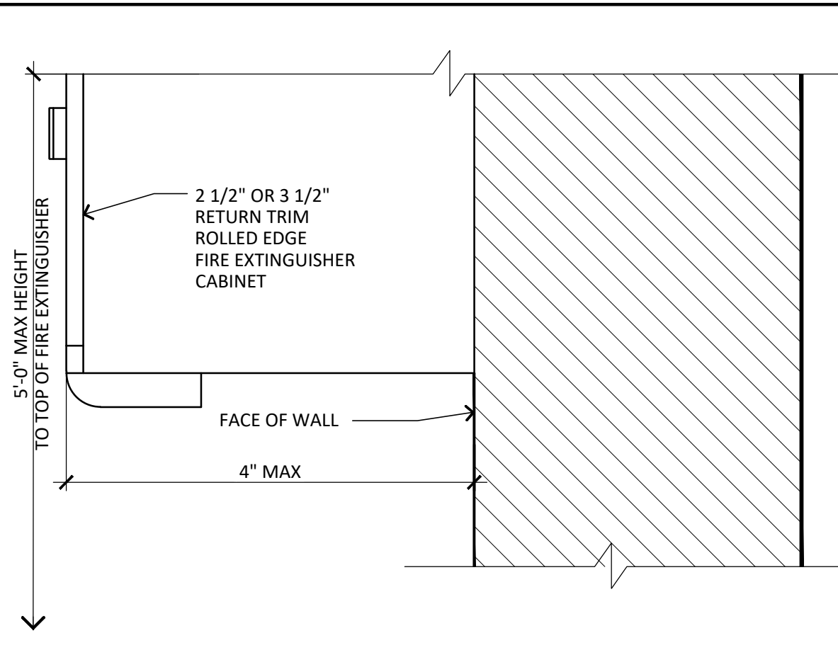
1 SURFACE MTD. FIRE EXTINGUISHER CAB. SCALE: N.T.S.
