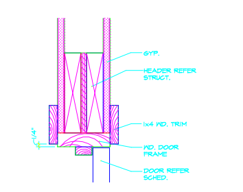
04 TYP. INTERIOR DOOR FRAME 3" x 1'-0"
