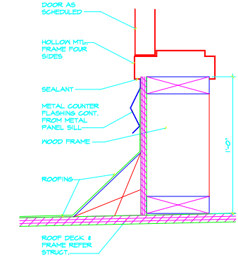
13 SILL DOOR 201 3" x 1'-0"
