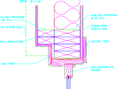
06 JAMB WINDOW A-1 3'1"-0"
