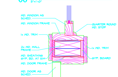
10 JAMB DOOR 101, WIN A-1 3'1"-0"
