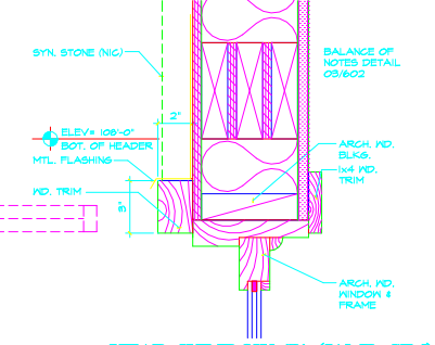
01 HEAD WINDOW 'B' (JAMB SIM) 3'1"-0"
