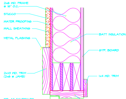
17 DOOR HEAD 108A (JAMB SIM) 3'1"-0"
