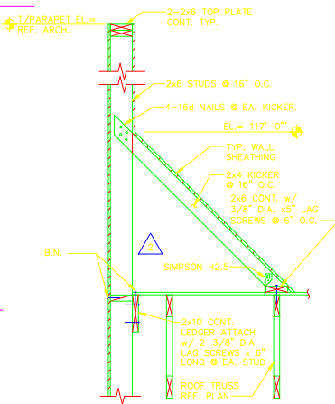
13 SECTION SCALE: 3/4"=1'-0"
