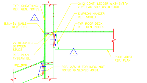
10 SECTION SCALE: 3/4"=1'-0"
