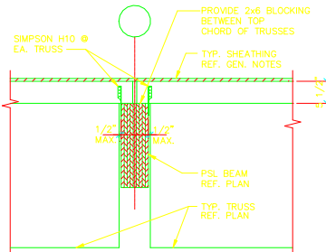
8 SECTION SCALE: 3/4"=1'-0"
