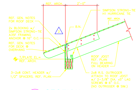
11 SECTION SCALE: 3/4"=1'-0"
