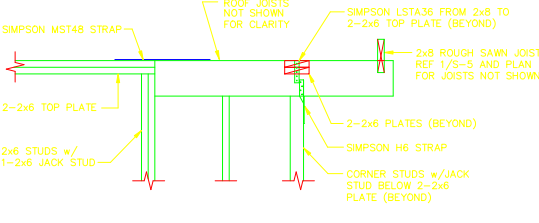
15 SECTION SCALE: 3/4"=1'-0"
