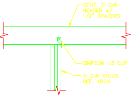
12 SECTION SCALE: 3/4"=1'-0"
