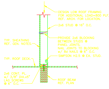
9 SECTION SCALE: 3/4"=1'-0"
