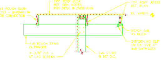
14 SECTION SCALE: 3/4"=1'-0"
