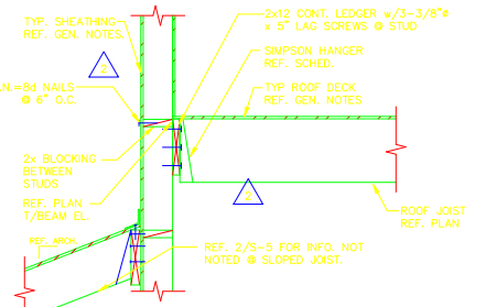
10 SECTION SCALE: 3/4"=1'-0"
