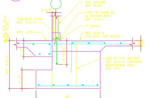
17 SECTION SCALE: 3/4"=1'-0"
