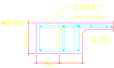
19 SECTION SCALE: 3/4"=1'-0"
