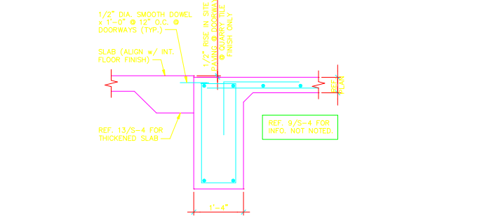
14 SECTION SCALE: 3/4"=1'-0"
