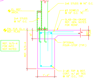
16 SECTION SCALE: 3/4"=1'-0"
